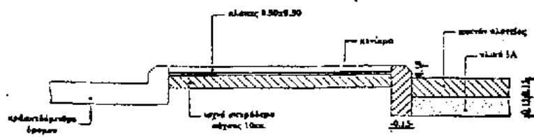
ΤΟΜΗ Α-Α
