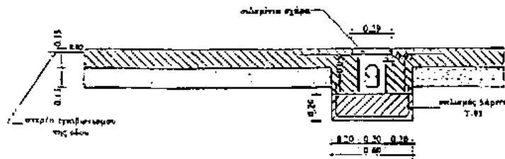
ΤΟΜΗ Β-Β
