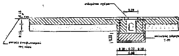
ΤΟΜΗ Β-Β
