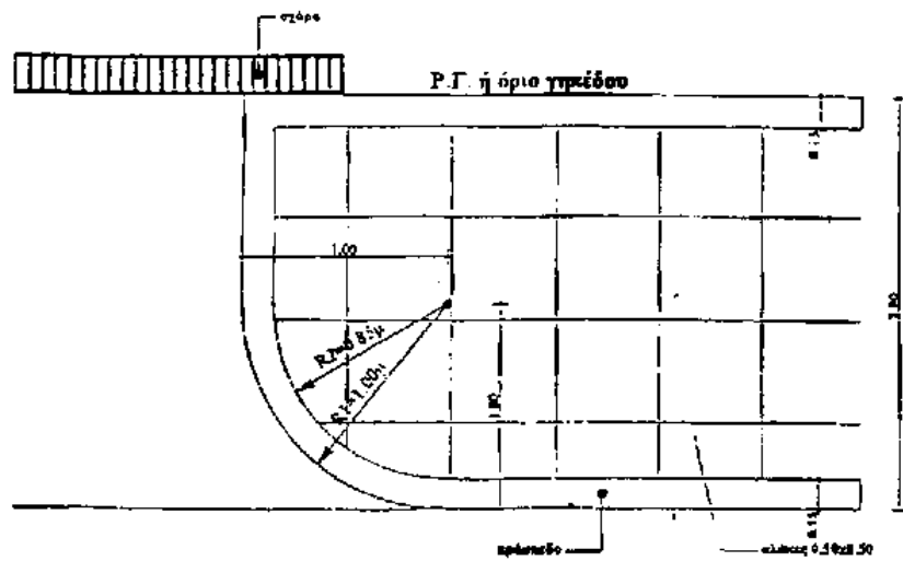
ΚΑΤΟΨΗ 1.15
