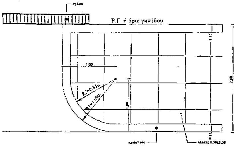
ΚΑΤΟΨΗ 1:25
