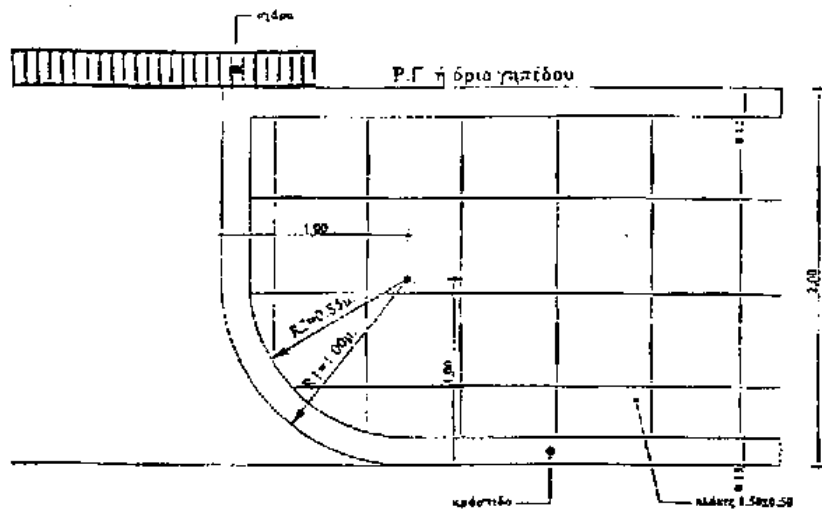
ΚΑΤΟΨΗ 1:25
