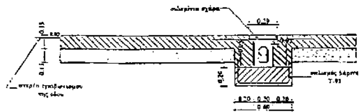
ΤΟΜΗ Β-Β
