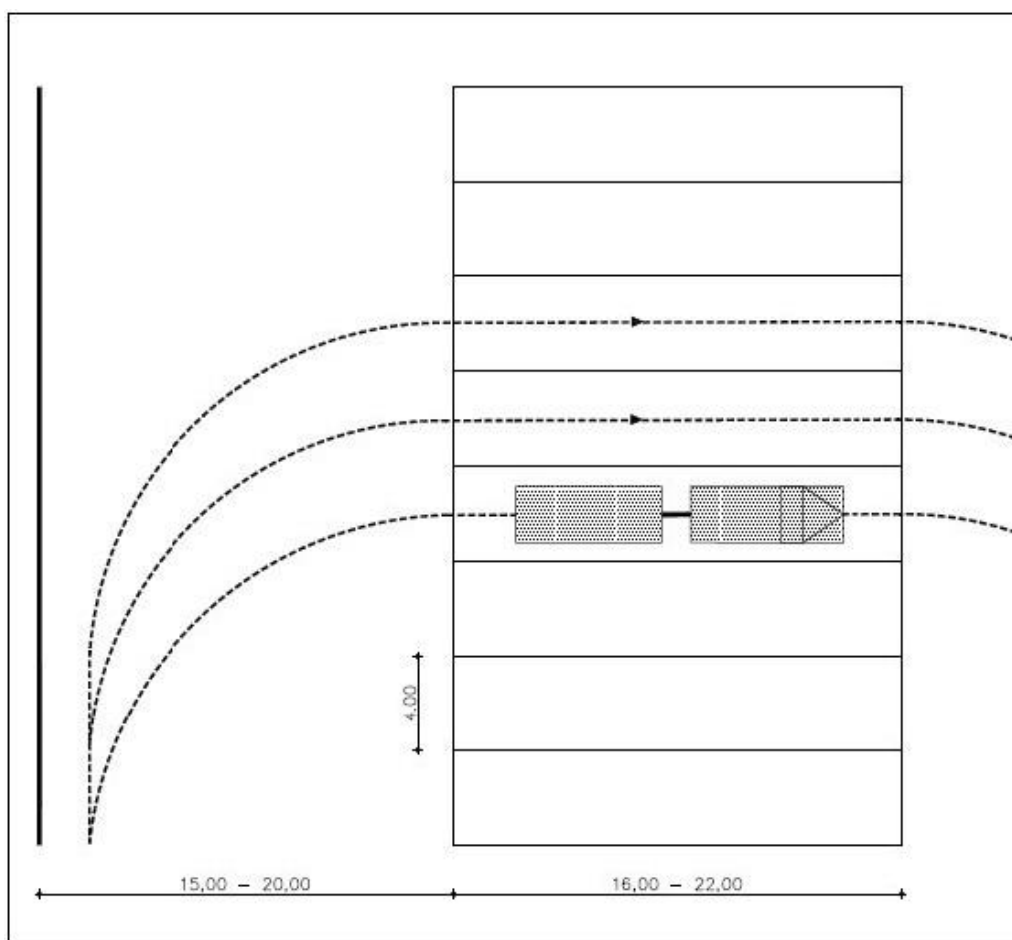
Σχήμα 8 Στάθμευση αρθρωτών λεωφορείων σε κλίση 90°
