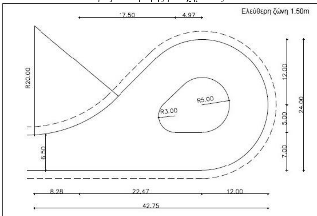
Σχήμα 2 Χώρος αναστροφής για όχημα έως 6m
