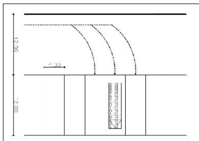
Σχήμα 7 Στάθμευση λεωφορείων σε κλίση 90°
